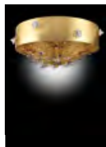
099/4S Ø 60 h. 31 Oro foglia 4 x E27 max 42W
