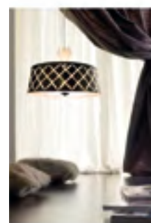
073/3S ø 40 x h. 34 Bianco vetro nero 3 x E27 max 42W
