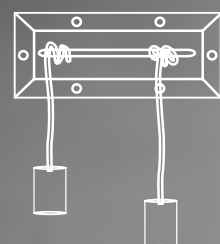
SERIE RETRO' ART. 1201A2 L. 33X13.5 SP. 10.5 H REGOLABILE COLORE FERRO NATURALE 2XE27 MAX 70 W
