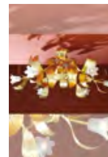
089/6PL Ø 88 h. 37 Plafoniera Oro foglia 6 x G9 max 33W
