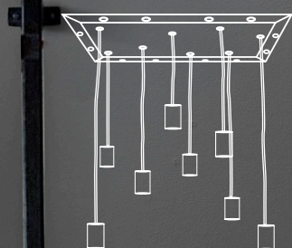
SERIE RETRÒ ART. 12018S L. 34X64 H REGOLABILE COLORE FERRO NATURALE ORO FOGLIA 8XE27 MAX 70W
